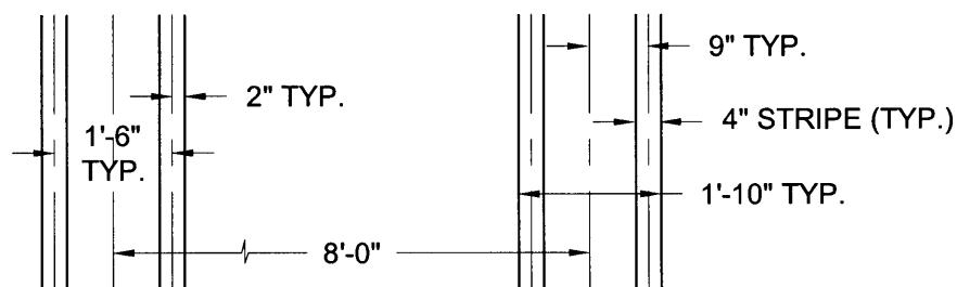
DETAIL A-A
