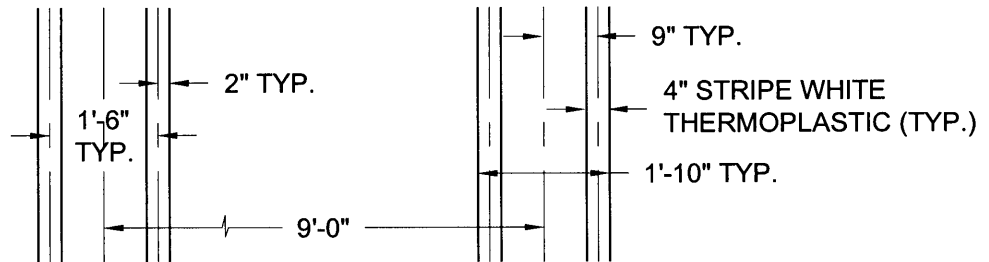
DETAIL A-A
